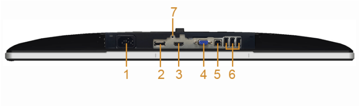
無顯示器支架的底視圖
